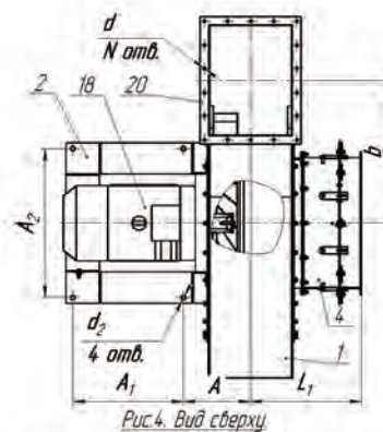
Рис.4. Вид сверху.
